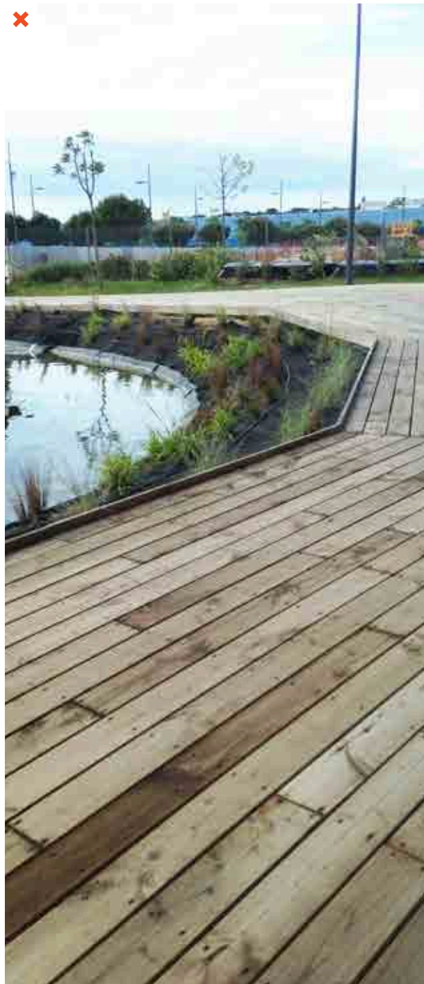
Exemple d'un platelage bois lisse et en pente pouvant devenir glissant. ©AQC
