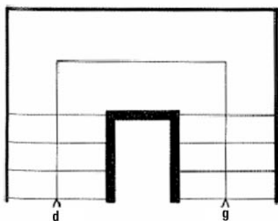
Escalier avec un grand palier de repos en fond de cage.
