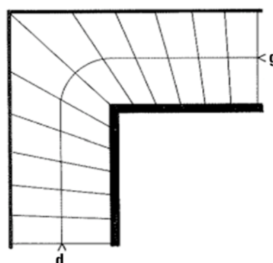
Escalier balancé dans une cage parallèle et rectangulaire avec une seconde volée d'équerre (quart tournant)
