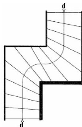
Escalier à deux coudes inversés
