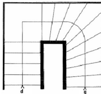
Escalier mixte avec un palier de repos et des marches balancées.
