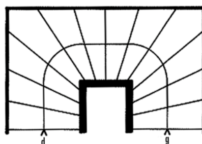
Escalier à trois volées d'équerre, avec un jour central (deux quarts tournant)
