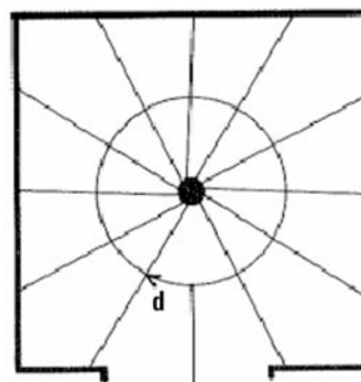
Escalier à vis dans une cage carrée
