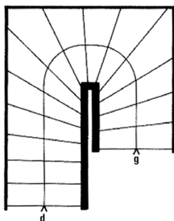
Escalier à trois volées d'équerre, avec un jour central (deux quarts tournant)
