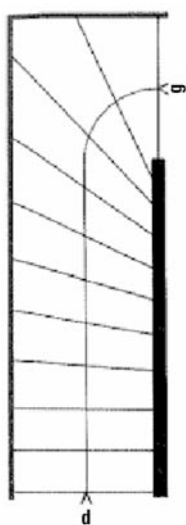
Escalier balancé dans une cage parallèle et rectangulaire
