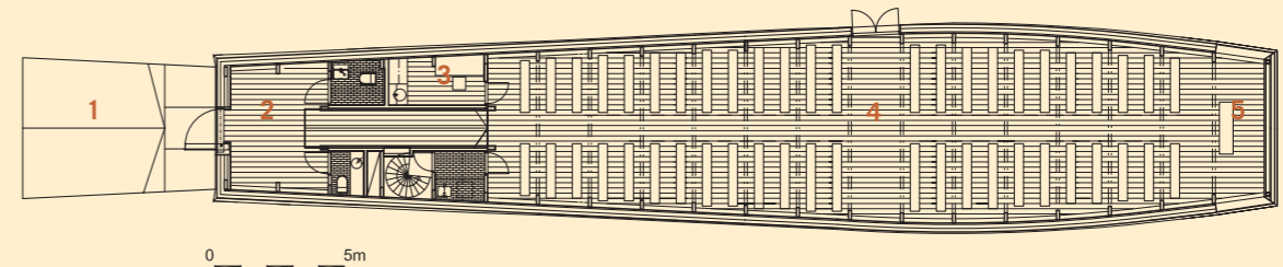
▲ Plan : 1- Parvis, 2- Vestibule, 3- Sacristie, 4- Nef, 5- Chœur.
